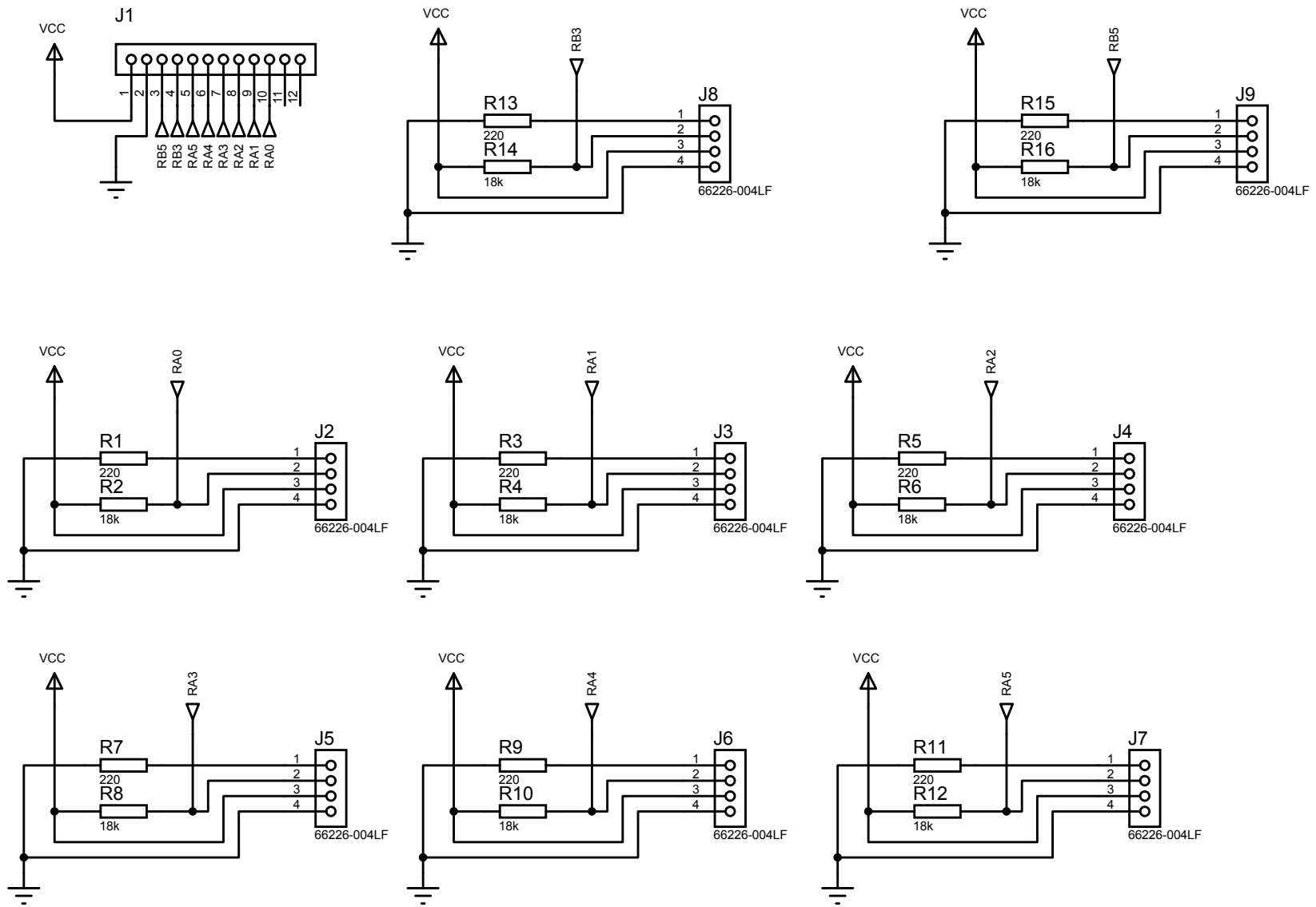
Módulo CNY70 2.1 - Placa de sensores
